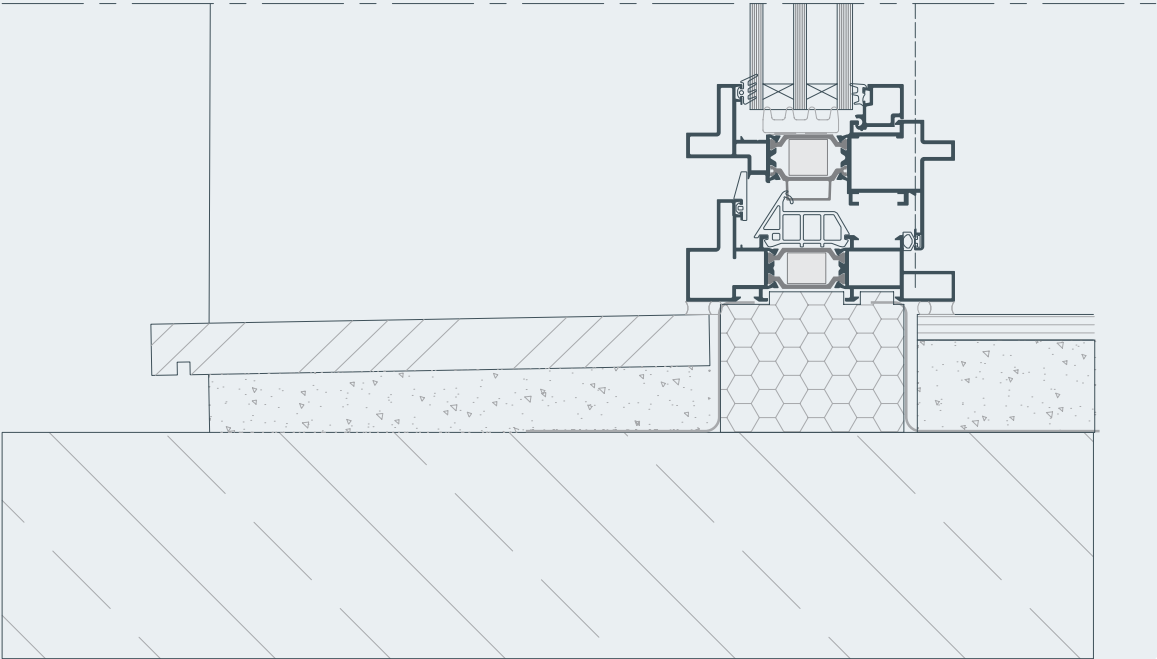
Secțiune inferioară B
