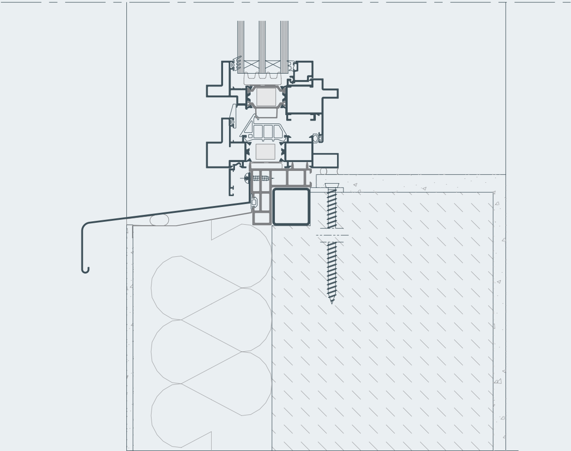
Secțiune inferioară A
