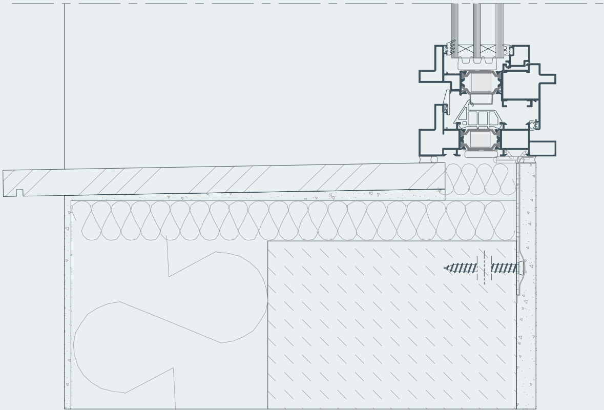
Secțiune inferioară A
