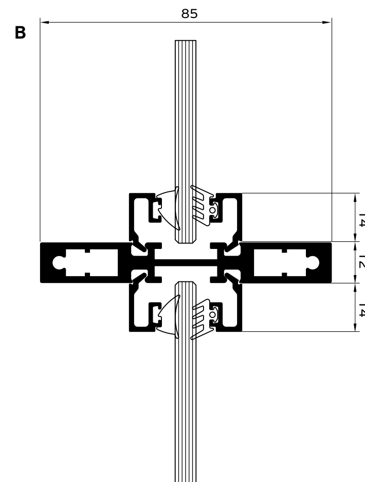
Vertikalno nadsvetlo
