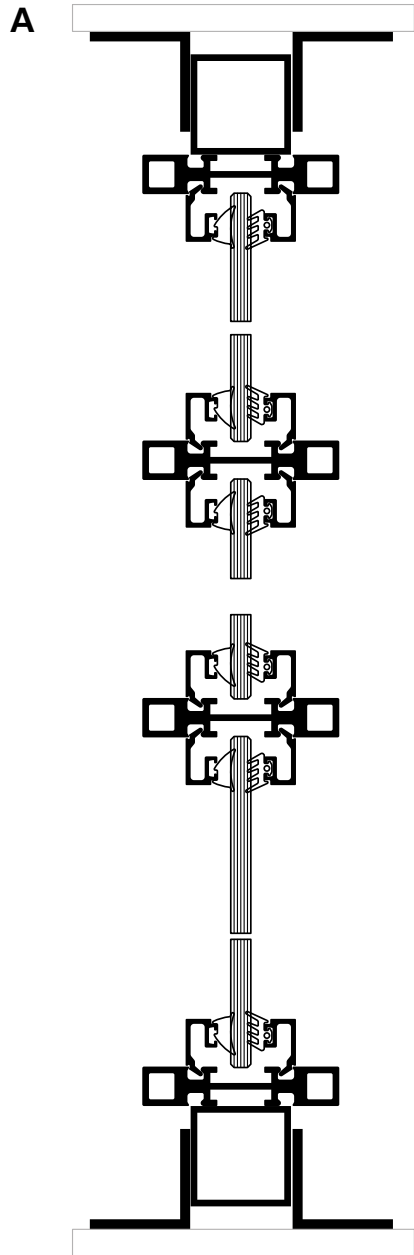
Secțiune verticală
