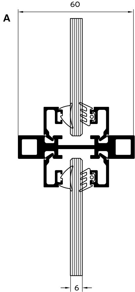
Traversă (dispunere pe orizontală)
