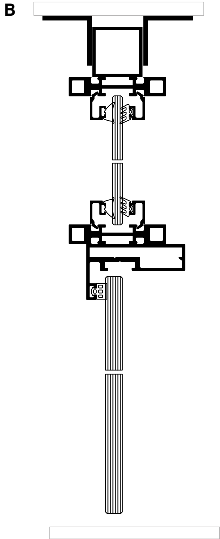
Secțiune verticală a ușii cu supralumină
