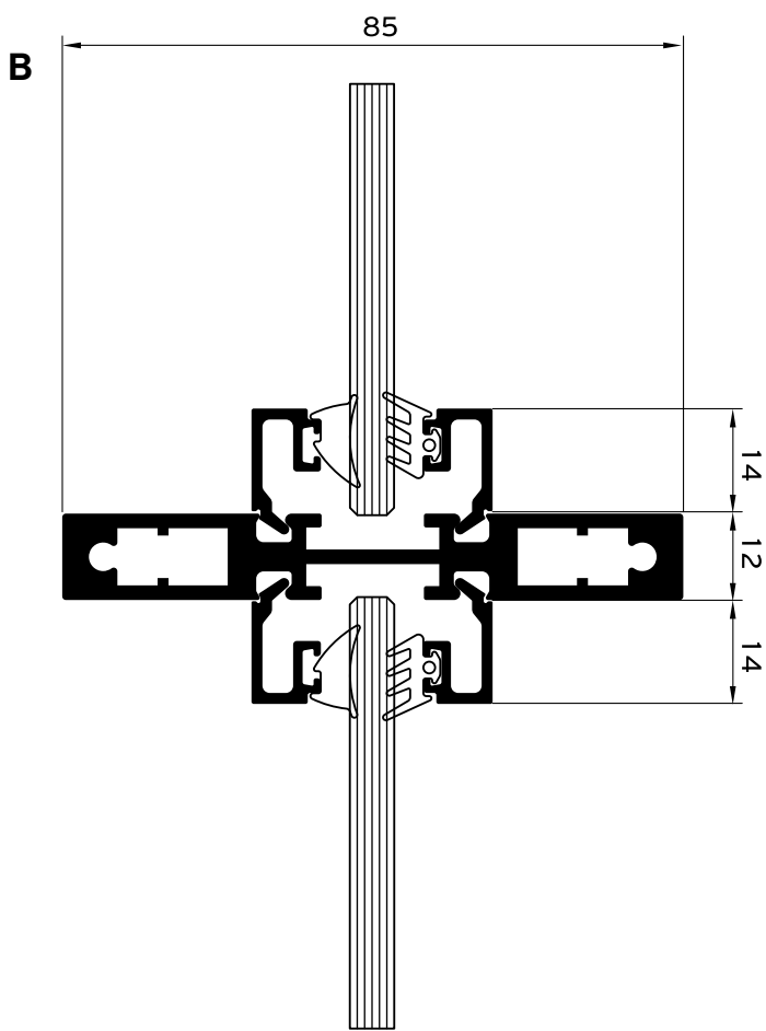
Montant (dispunere pe verticală)
