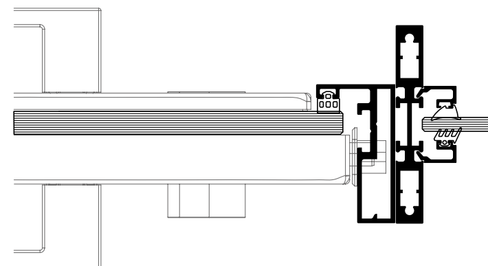
DETALIU BROASCĂ
