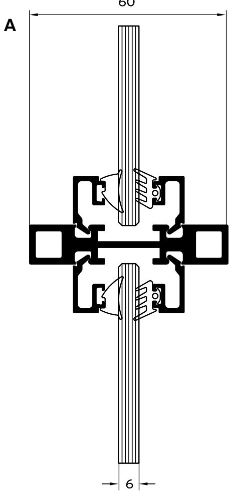
Οριζόντια τραβέρσα
