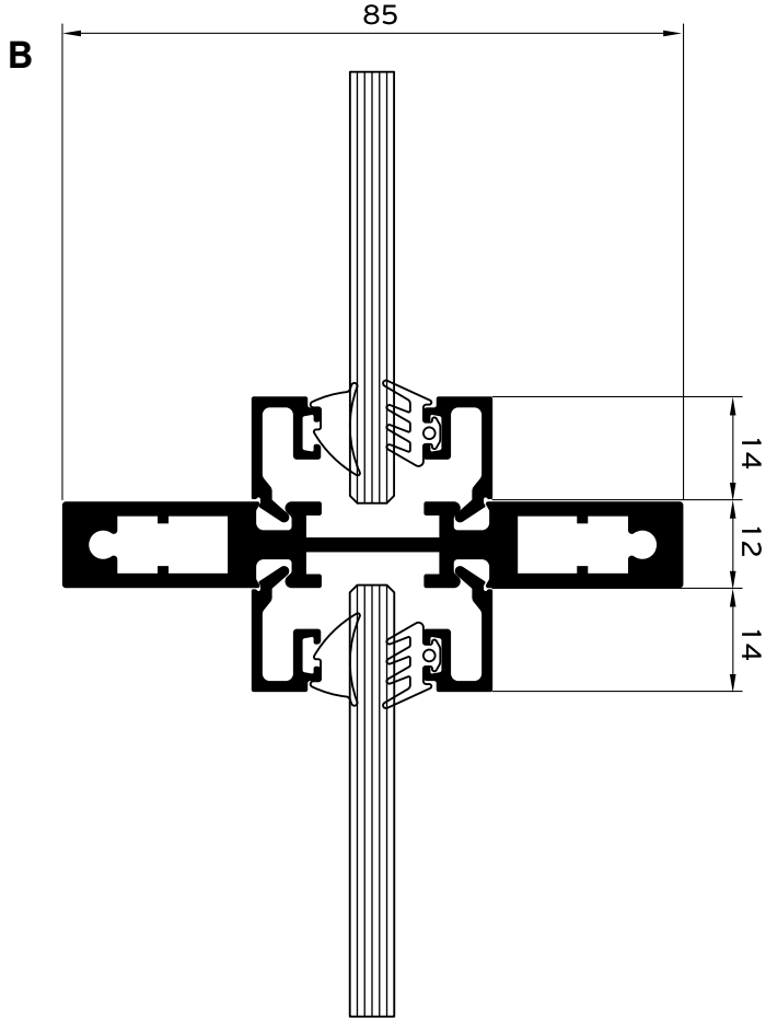
Κατακόρυφη τραβέρσα
