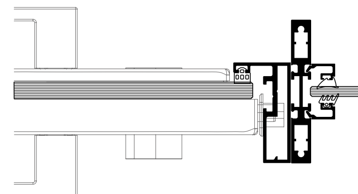
ΛΕΠΤΟΜΕΡΕΙΑ ΚΛΕΙΔΩΜΑΤΟΣ
