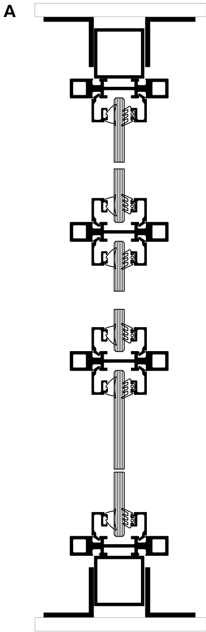
Κάθετη τομή τριπλό
