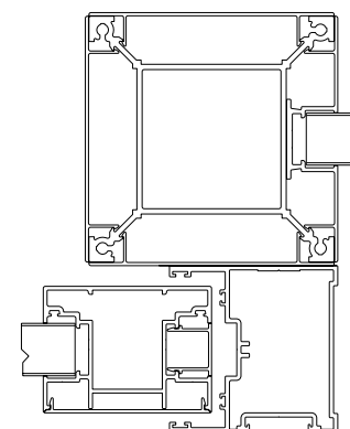
Κλείσιμο αυλόπορτας
