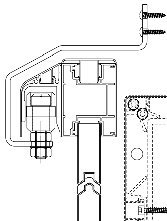
Μηχανισμός (άνω)
