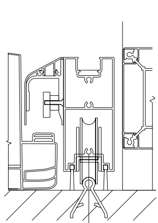
Μηχανισμός (κάτω)
