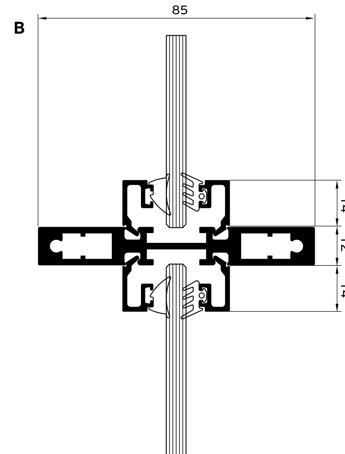
Vertikalno nadsvetlo
