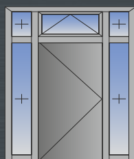
Usa intr-un canat mobil placat cu panel izolan, supralumina si laterale fixe
