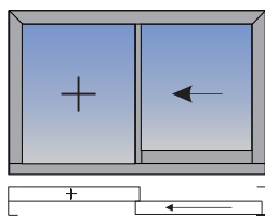
Rrëshqitje majtas me pjesë fikse nga jashtë
