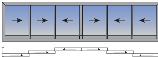
6 kanata rrëshqitëse me takim kokë më kokë (Tipi i takimit nga brenda)
