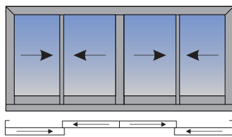
Rrëshqitje paralele me 4 kanata takim kokë më kokë (Tipi i takimit nga jashtë)
