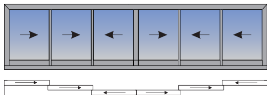
6 kanata rrëshqitëse me takim kokë më kokë (Tipi i takimit nga jashtë)
