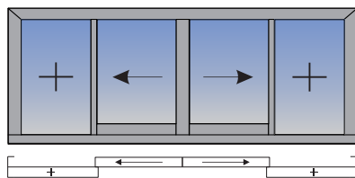
Rrëshqitje me takim kokë më kokë me 2 kanata dhe 2 pjesë fikse
