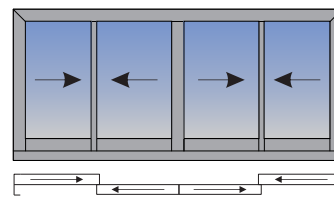
Rrëshqitje paralele me 4 kanata takim kokë më kokë (Tipi i takimit nga brenda)
