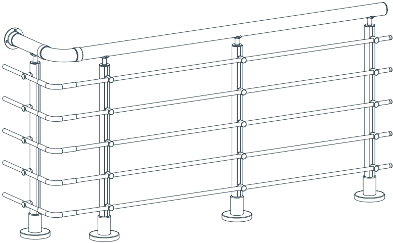
Στρογγύλα προφίλ και οριζόντιες μπάρες Round profiles and horizontal bars
